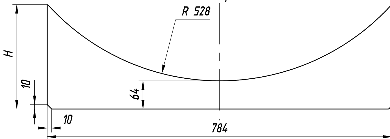
Рис. 3 (1:5)
